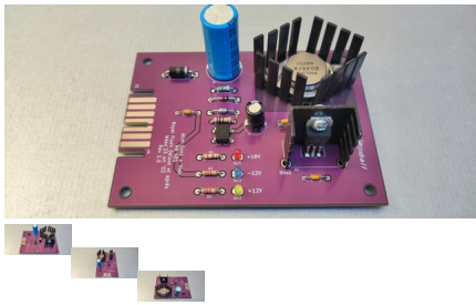
Carte régulation MA481
